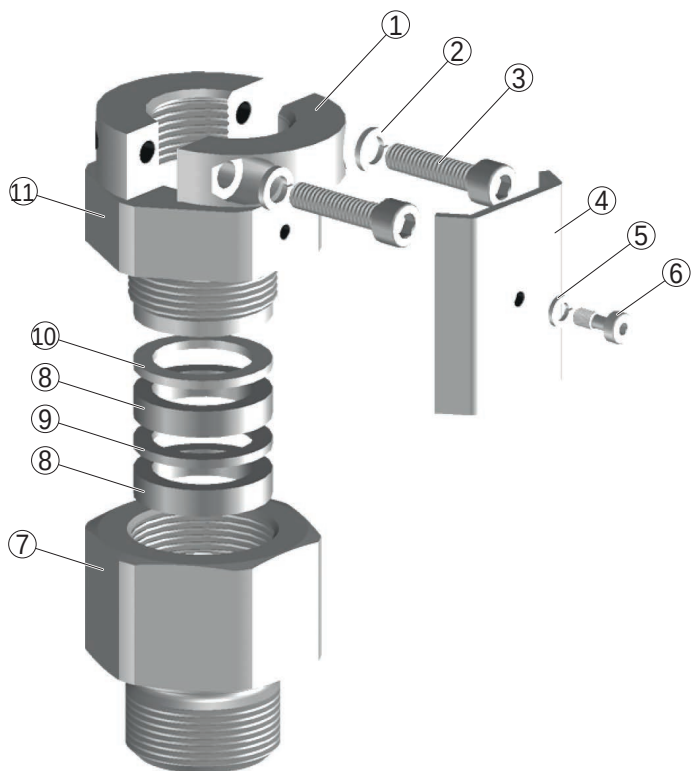
插图. 1: ARV 200 - 至16 bar (232 psig)
