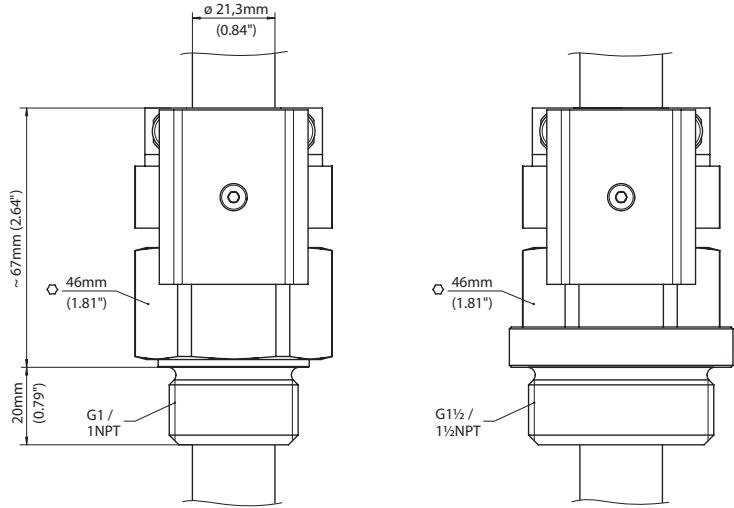
插图. 2: 制动螺旋接头ARV 200 , 至 16 bar (232 psig) , 用于 SITRANS LVL200E
